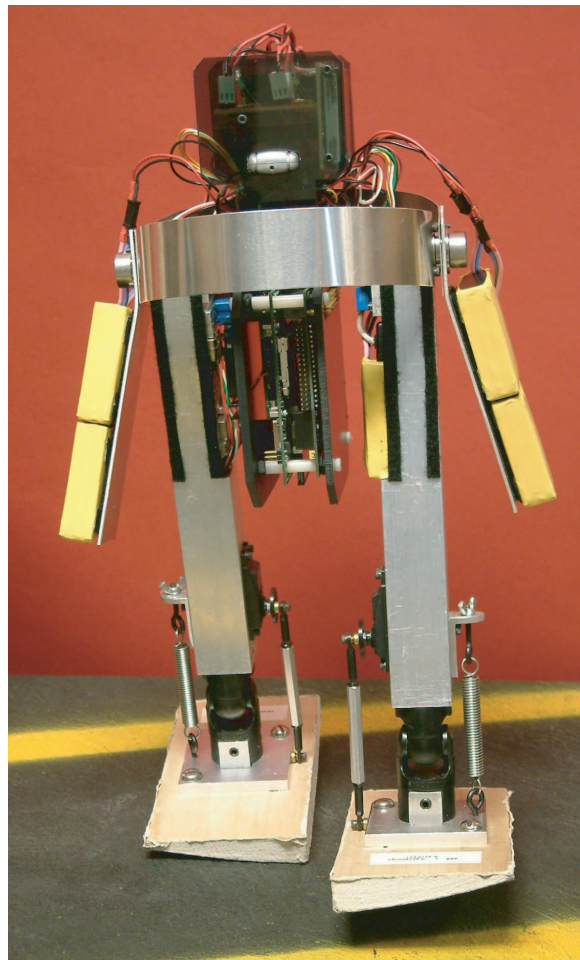
Figure 3: The MIT learning biped
